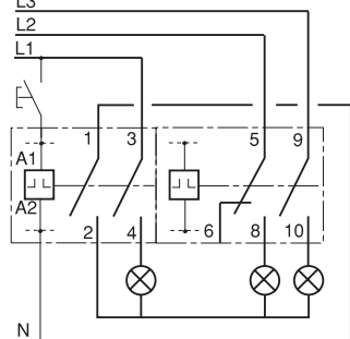
Импульсное реле TL 16 А с ETL, 3 полюса + нейтраль
