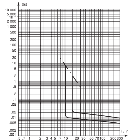
NG125, кривая MA
