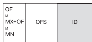
OF Блок-контакт состояния MX Независимый расцепитель MN Расцепитель минимального напряжения OFS Блок-контакт ID Дифференциальный выключатель нагрузки
