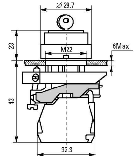
Переключатели XB4BG
