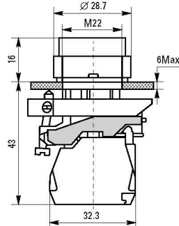
Кнопки XB4BL
