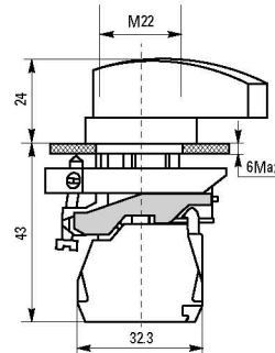
Переключатели XB4BJ
