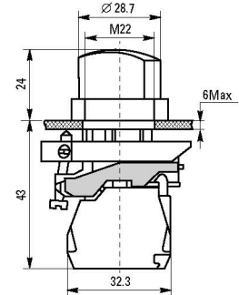
Переключатели XB4BG
