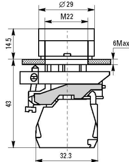
Кнопки XB4BW3
