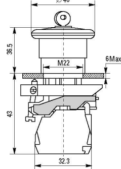
Переключатели XB4BJ
