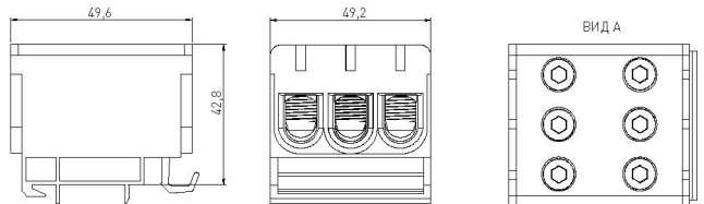
КСВ 16-50 (тройные)
