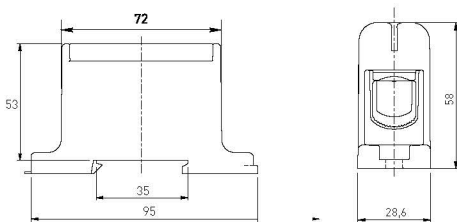
КСВ 35-240
